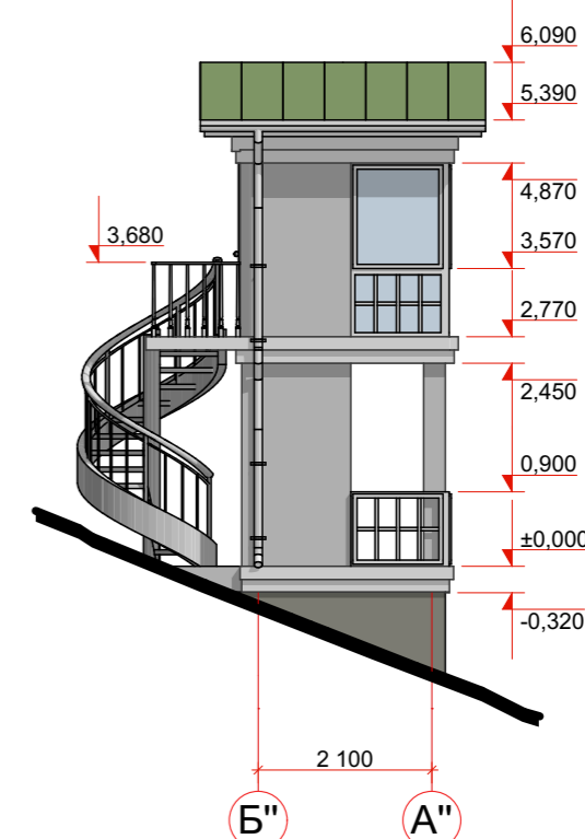
Фасад в осях Б-А. М 1:100
