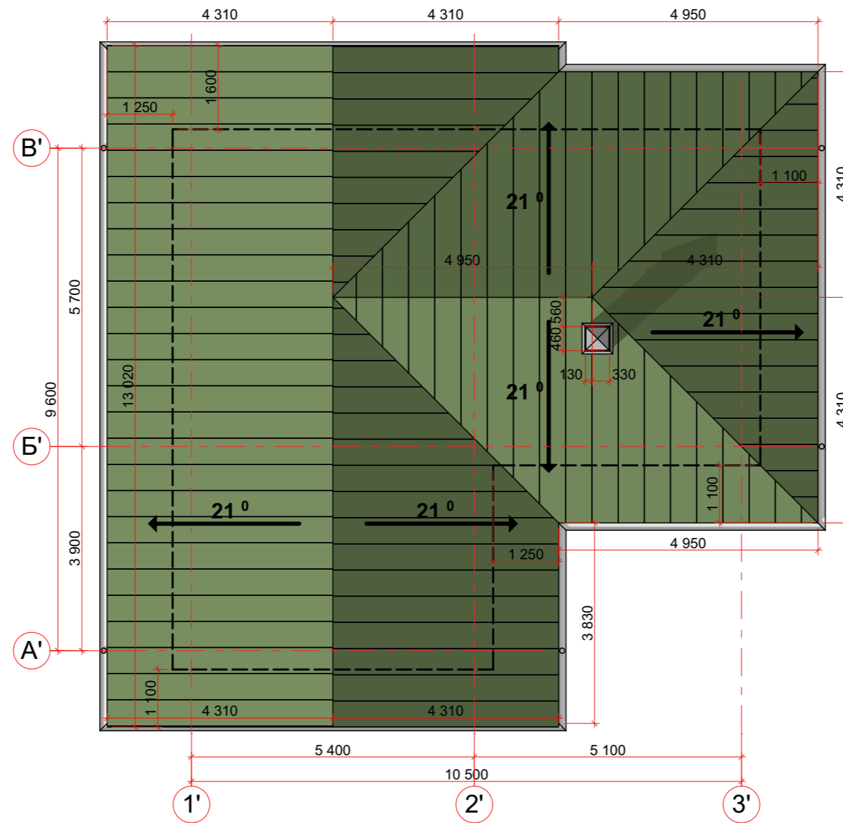
План кровли. М 1:100
