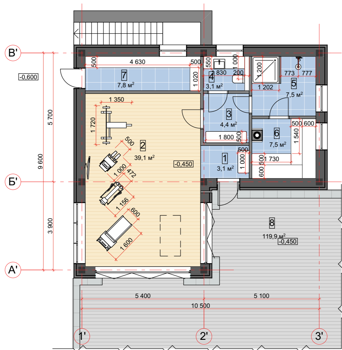
План 1-го этажа с расстановкой мебели М 1:100
