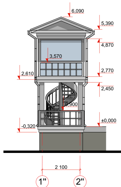
Фасад в осях 2-1. М 1:100
