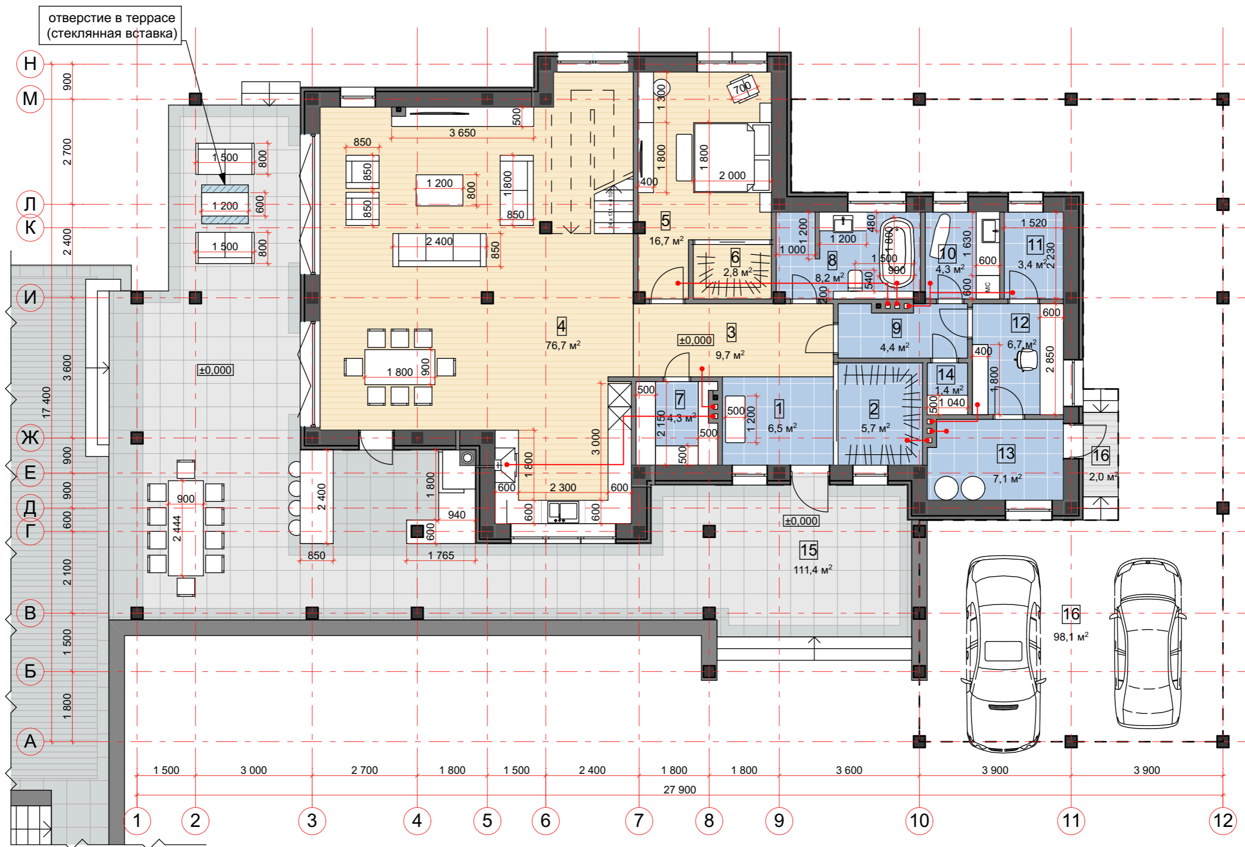
Экспликация помещений 1-го этажа
