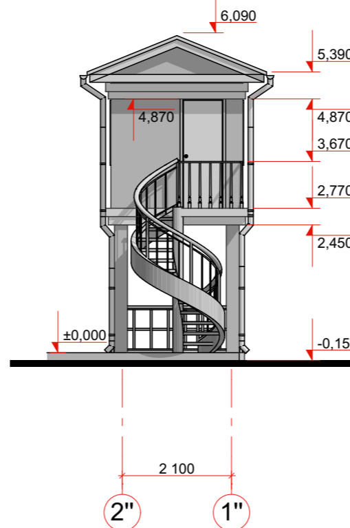
Фасад в осях 2-1. М 1:100
