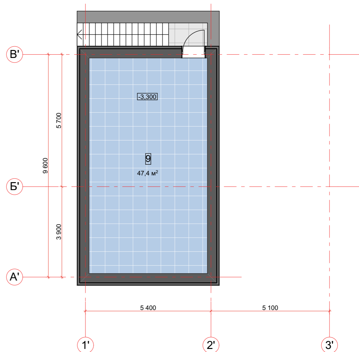
План цокольного этажа М 1:100
