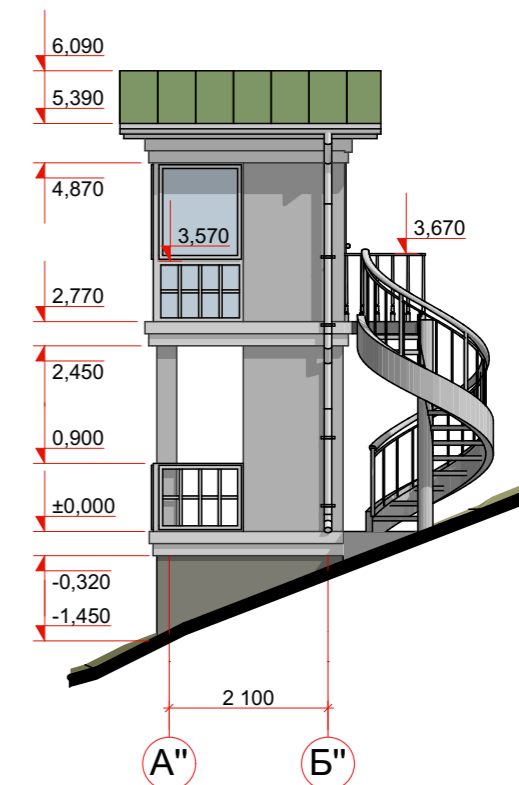
Фасад в осях Б-А. М 1:100
